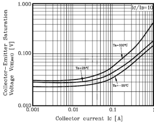
Fig. 5 I_C - V_{CE}
