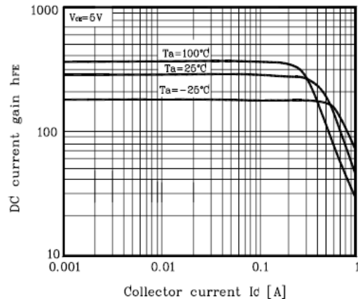
Fig. 6 h_{FE} - I_C
